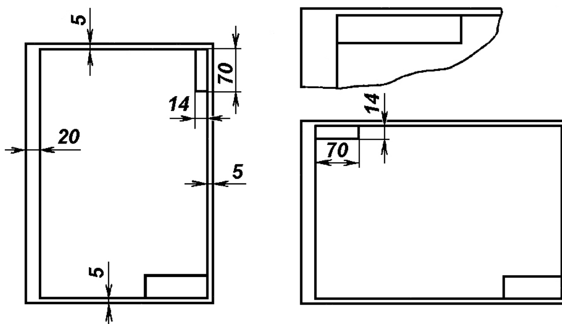
Рамки поля чертежа
